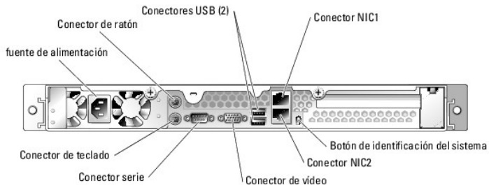
Figura 1-2. Características e indicadores del panel posterior
